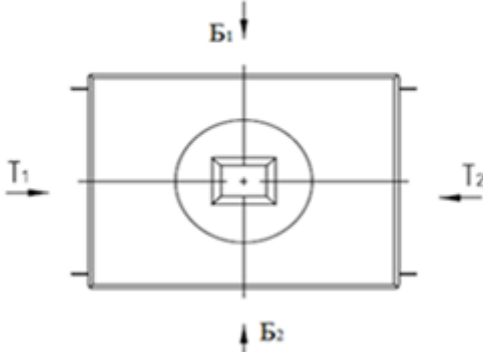
Схема обозначения сторон ККС 2,5-10(80) СУ-ССД-Пайп (вид сверху)
