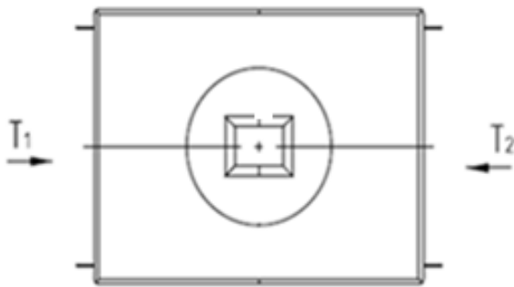
Схема обозначения сторон ККС 1-10(80) СУ-ССД-Пайп (вид сверху)
