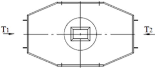
Схема обозначения сторон ККС 3,5-10(80) СУ-ССД-Пайп (вид сверху)
