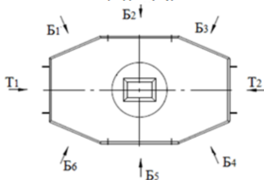
Схема обозначения сторон ККС 4-10(80) СУ-ССД-Пайп (вид сверху)
