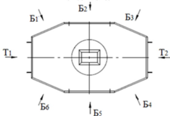
ТЗ на предустановку муфт в стенки колодца ККС 5-10(80) СУ-ССД-Пайп*
