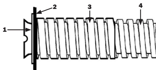
Рисунок 9.11 – Ввод трубы «ССД-Пайп» в полимерный колодец
