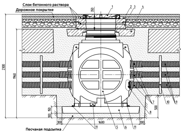
Рисунок Г.15 – Схема установки кабельного колодца ККП-4-ССД на проезжей части улиц
