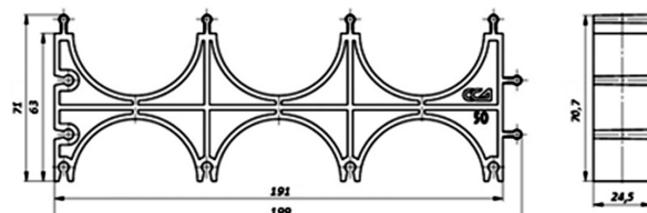
Кластер ССД-Пайп OD=50 мм тройной
