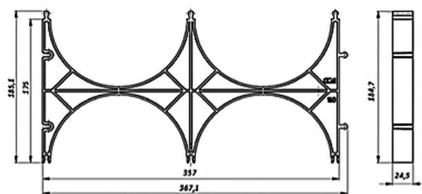
Кластер ССД-Пайп OD=160 мм двойной
