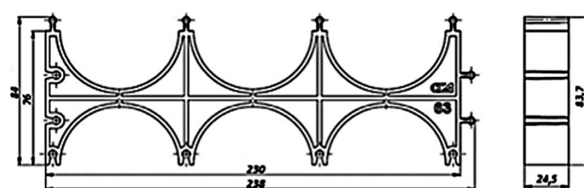
Кластер ССД-Пайп OD=63 мм тройной
