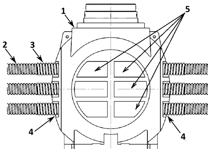
Рисунок 9.10 – Ввод труб «ССД-Пайп» в полимерный колодец ККП-4-ССД
