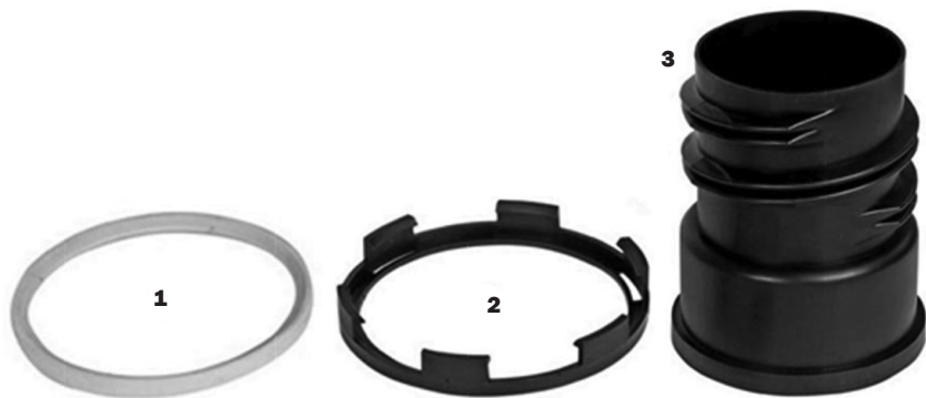
Рисунок 2.7 – Элементы переходной муфты 1 – уплотнительное кольцо; 2 – фиксатор кольца; 3 – корпус переходной муфты
