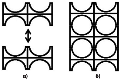
Рисунок 9.15 – Вертикальное соединение кластеров ССД а – направление соединения; б – блок из трёх кластеров, соединённых по вертикали
