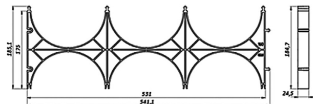
Кластер ССД-Пайп OD=160 мм тройной
