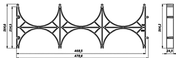
Кластер ССД-Пайп OD=140 мм тройной
