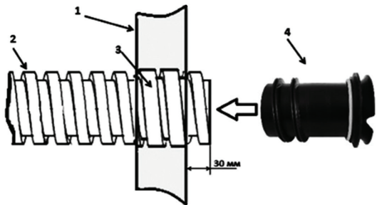
Рисунок 9.9 - Ввод короткого отрезка трубы в колодец через вмонтированную муфты 1 – наружная поверхность стены колодца; 2 – короткий отрезок трубы (1 или 1,5 м); 3 – отрезок соединительной муфты, вмонтированный в стену колодца; 4 – внутренняя заглушка, вкручиваемая в трубу
