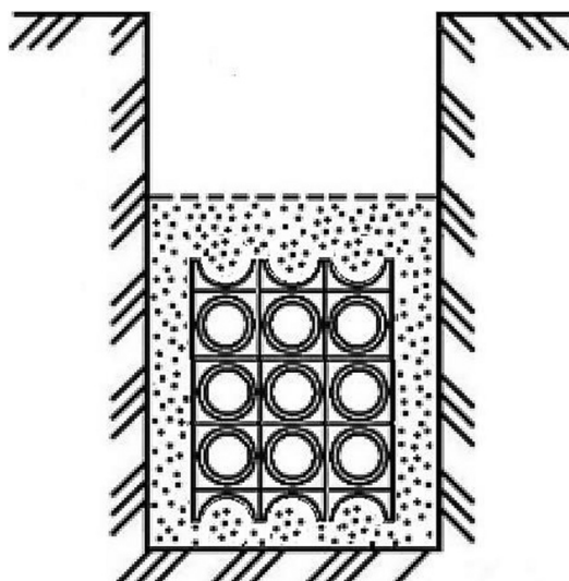
Рисунок Б.2 – Блок труб «ССД-Пайп» в траншее.
