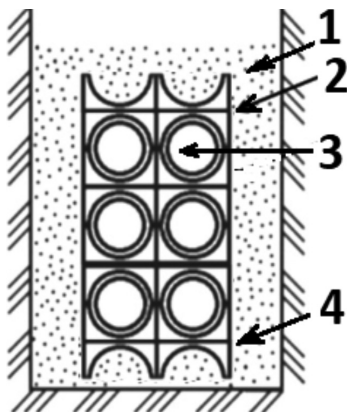
Рисунок 9.16 – Положение труб в блоке кластеров 1 – траншея с засыпкой; 2 – кластер, фиксирующий верхний ряд труб; 3 – трубы верхнего ряда; 4 – кластер, фиксирующий нижний ряд труб
