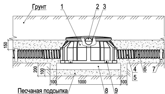
Рисунок Г.1 – Схема установки камеры оптической КОТ-1-ССД
