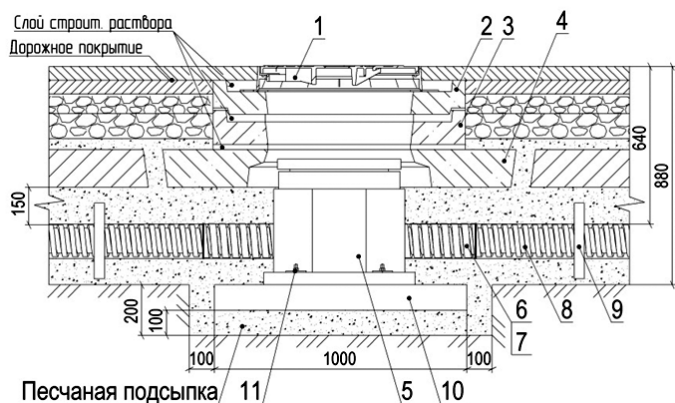
Рисунок Г.11 – Схема установки кабельного колодца ККП-1-ССД
