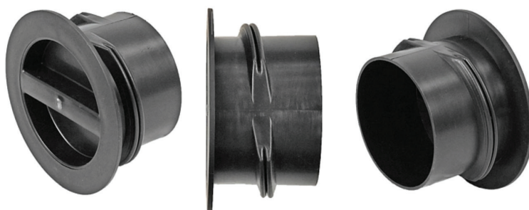
Рисунок 2.5 – Заглушки внутренние резьбовые для муфт, вмонтированных в стены колодцев «ККС-ССД-Пайп»
