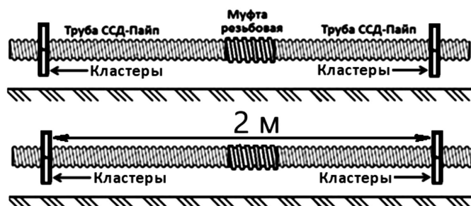
Рисунок 9.13 – Расстояние между блоками кластеров в траншее
